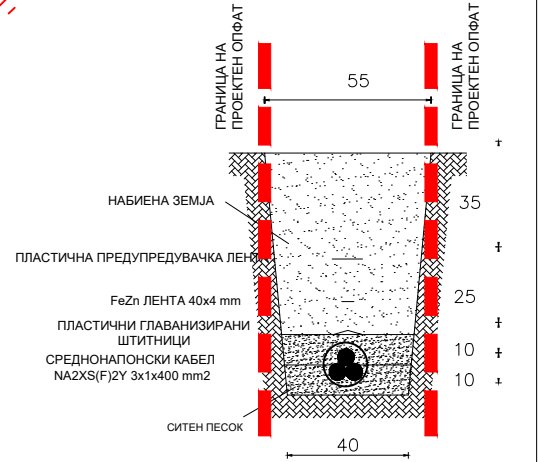
ПРИКАЗ НА КАБЕЛСКИ РОВ ЗА СН КАБЕЛ -ПРЕСЕК -
